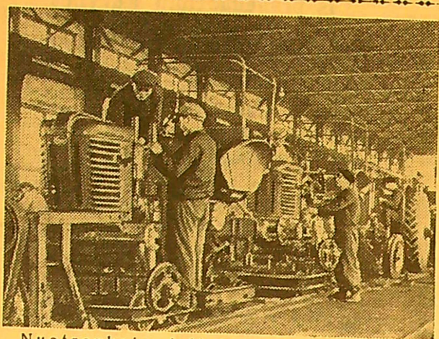
Nuotraukoje: traktorių surinkimas Kijano mašinių gamyklos ceche. Chan Con Siko nuotr. KLDK Centrinės telegramų agentūros fotokronika
