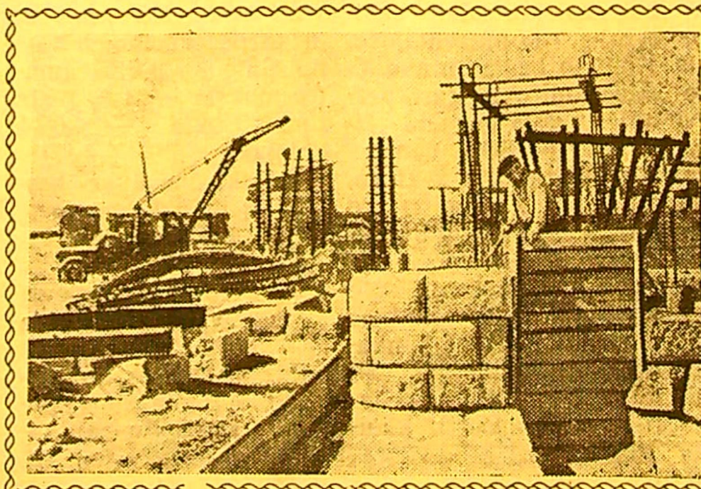
KIRGIZIJOS TSR. Seštojo penkmečio metais turi būti užbaigta Didžiojo Cujos kanalo statyba. Jo pagalba bus sudrėkinta 115 tūkstančių hektarų žemės Cujos slėnyje. Dabar vyksta kanalo rytų atšakos pradinio įrenginio statyba.
