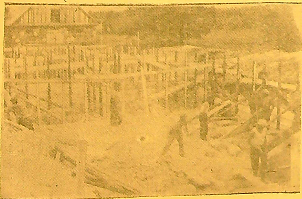
P. Cvirkos vardo kolūkyje Zarasų remonto-statybos kontora stato 500 tonų talpos silosą tranšėją.
