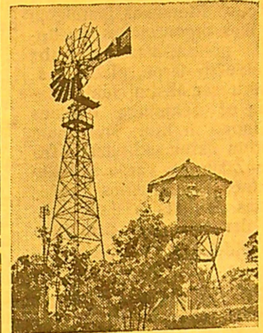
MASKVA. Visasąjunginė žemės ūkio paroda. Vėjo variklis „TV-8“ varoma vandens siurbkla.
