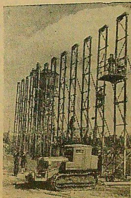
Novosibirskas. Statybos masinių gamyklai pavesta pagaminti Kulbiševu hidroelektrinės statybai stiebinų keltuvų partija.
